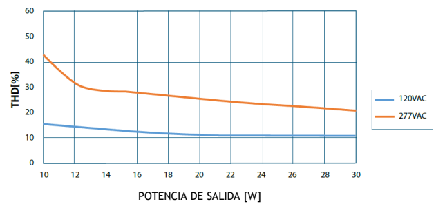
THD vs POTENCIA DE SALIDA
