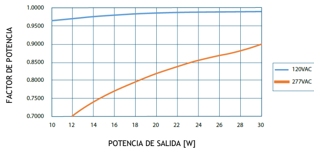
FACTOR DE POTENCIA vs POTENCIA DE SALIDA
