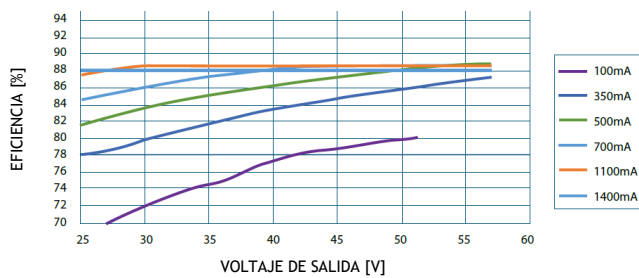
EFICIENCIA vs. VOLTAJE DE SALIDA (120VAC)
