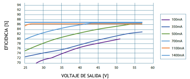
EFICIENCIA vs. VOLTAJE DE SALIDA (277VAC)
